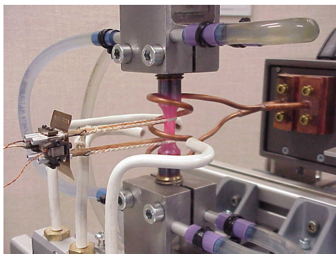
Indukcyjny system grzania próbek oraz komora kriogeniczna
