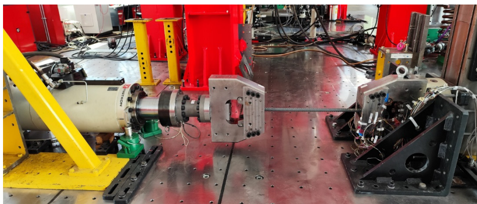
Serwocylinder hydrauliczny wraz z uchwytemi o nominalnym obciążeniu dynamicznym wynoszącym \pm 1000 kN
