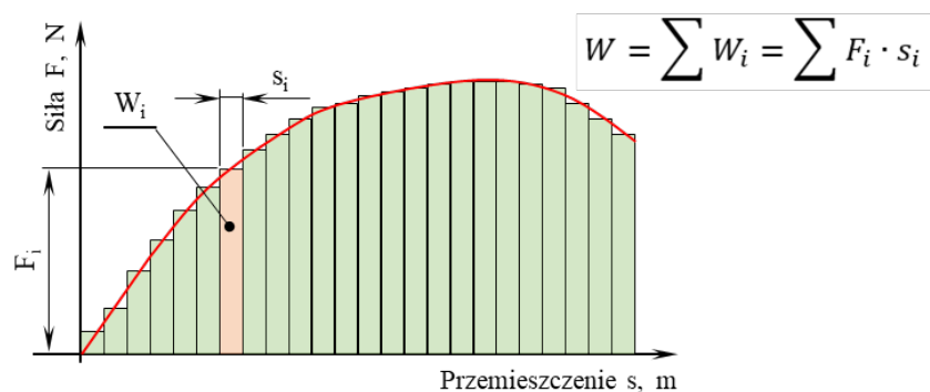
Rys. 5.5. Schemat wyznaczania pracy W prowadzącej do zniszczenia próbki
