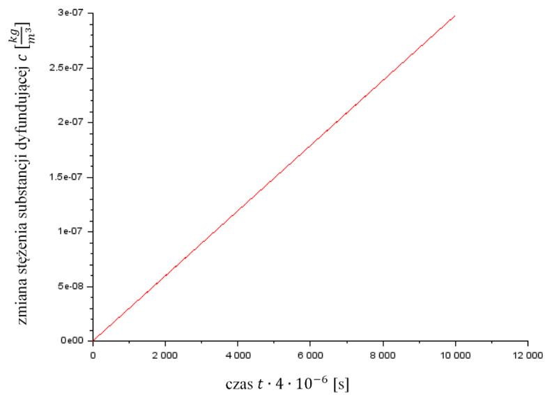
Rys. 6.62. Wykres zmian stężenia substancji dyfundującej na końcach wspornika przy źródle masy o wydajności 5 g/s
