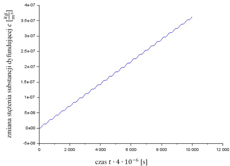
Rys. 6.31. Wykres zmian stężenia substancji dyfundującej w punkcie końcowym wspornika przy obciążeniu o wartości 200 kN
