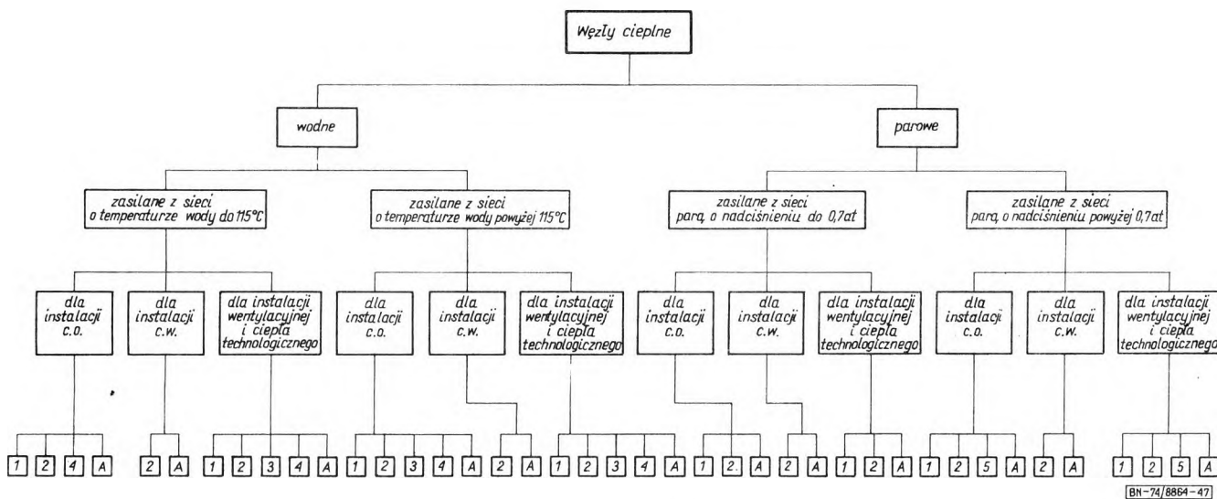
Schemat klasyfikacyjny węzłów ciepłnych
