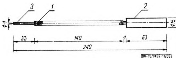
1 - odcinek z nawiniętym drutem, 2 - uchwyt, 3 - rdzeń
