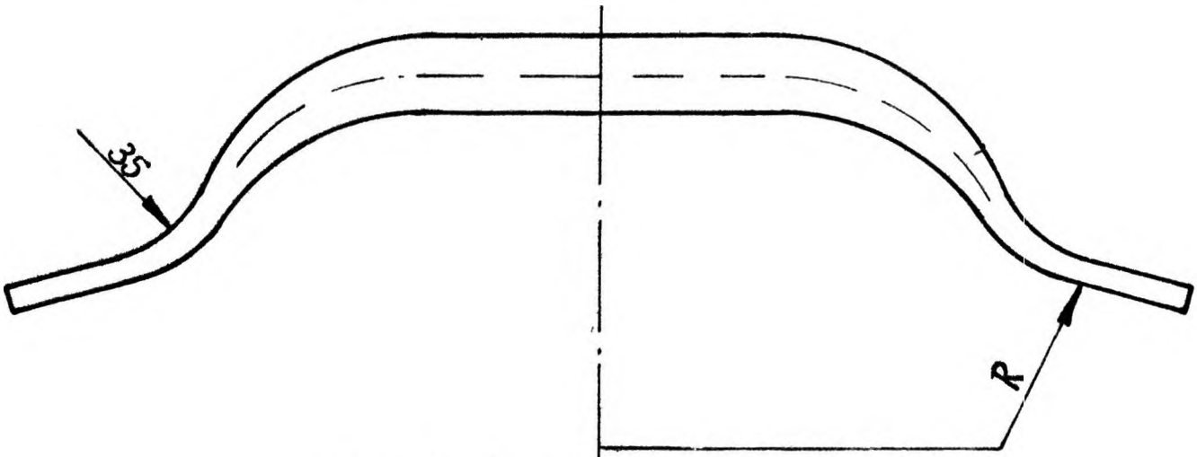
Rys. 4 Uchwyt typu III, odmiany B
