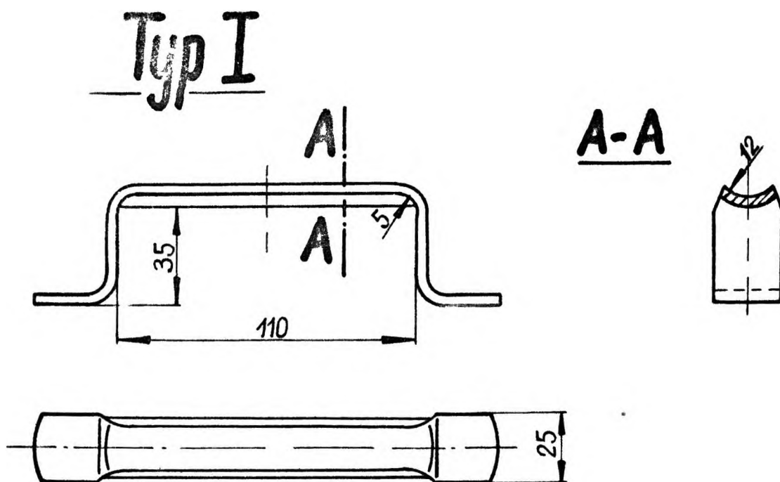
Rys. 1 Uchwyt typu I, odmiany A
