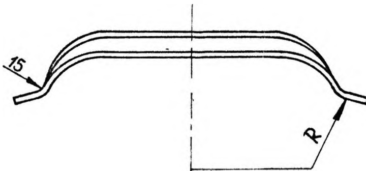
Rys. 5 Uchwyt typu III, odmiany A
