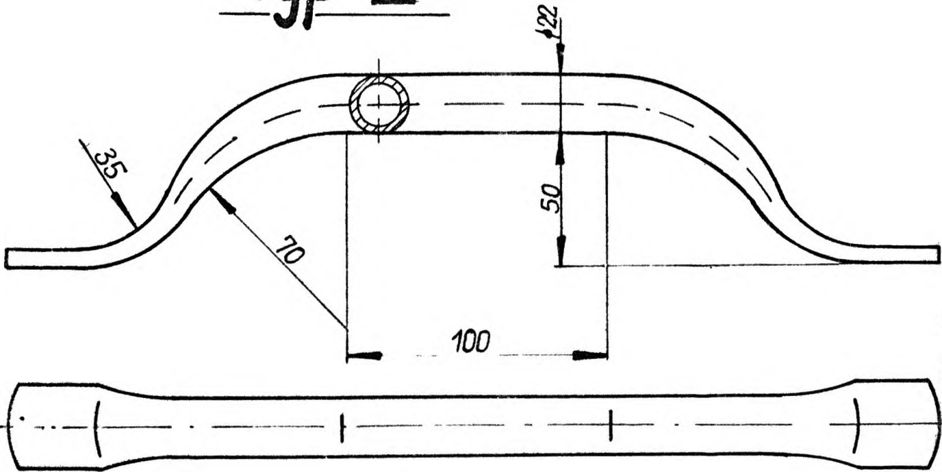
Rys. 3 Uchwyt typu III, odmiany A
