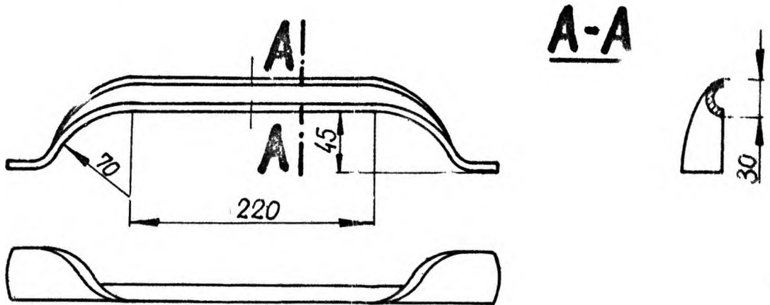
Rys. 5 Uchwyt typu III, odmiany A
