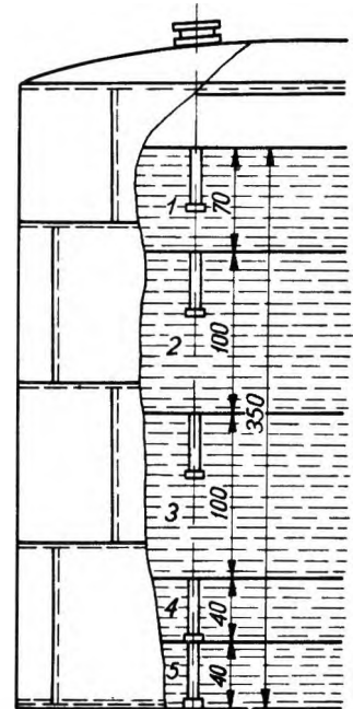
Rys. 3. Sposób pobierania próbek ze zbiorników stojących
