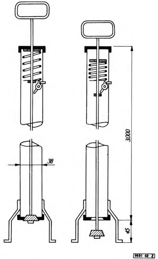
Rys. 2. Probnik rurowy
