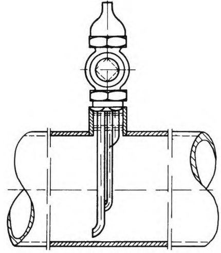
Rys. 4. Rurociągowy kurek spustowy
