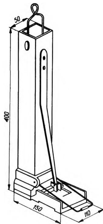
Rys. 1. Próbnik zatrząskowy
