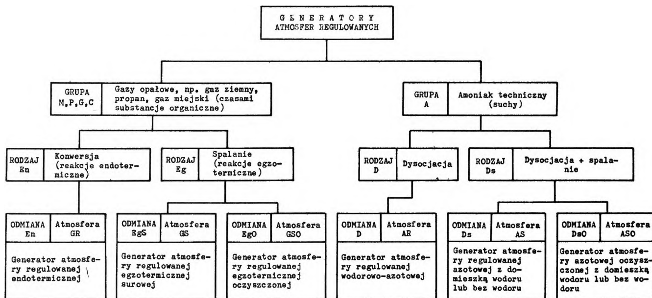
Rys. 2. Schemat klasyfikacyjny typowych generatorów atmosfer regulowanych
