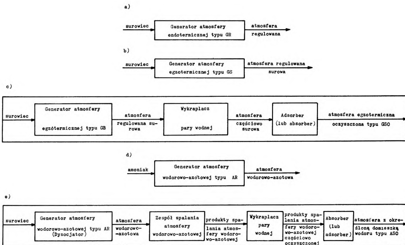
Rys. 1. Schematy blokowe typowych generatorów atmosfer regulowanych: a) generator atmosfery regulowanej endotermicznej, b) generator atmosfery regulowanej egzotermicznej surowej, c) generator atmosfery egzotermicznej oczyszczonej, d) generator atmosfery regulowanej wodorowo-azotowej z amoniaku, e) generator atmosfery regulowanej azotowej z amoniaku
